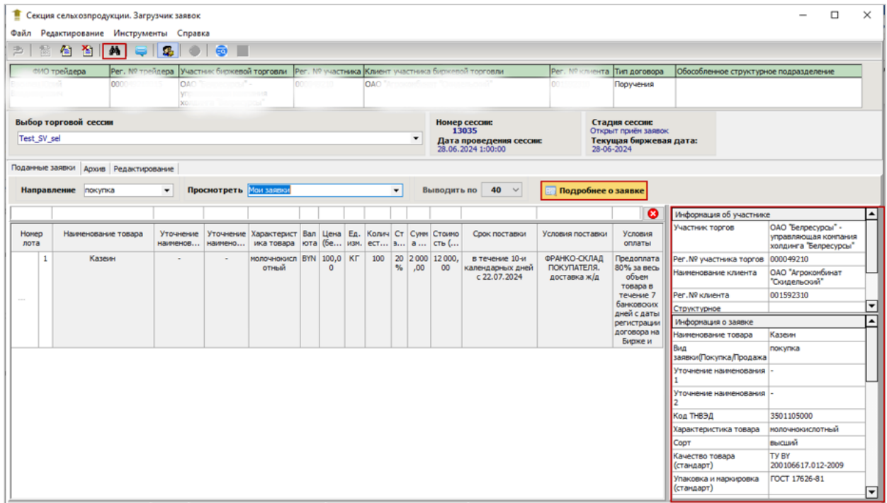
Рисунок 15 – Подробная информация о заявке
