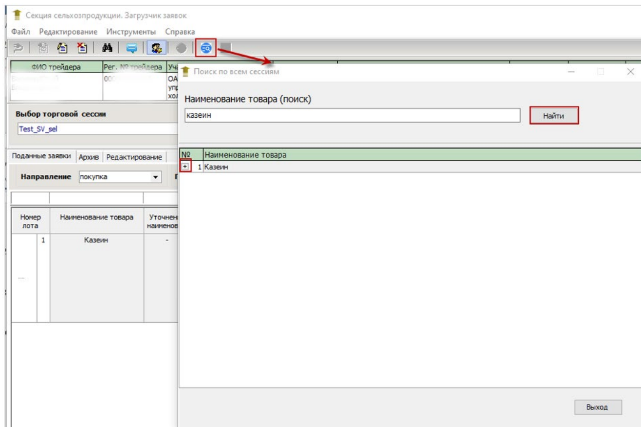
Рисунок 17 – Поиск товара по сессиям
