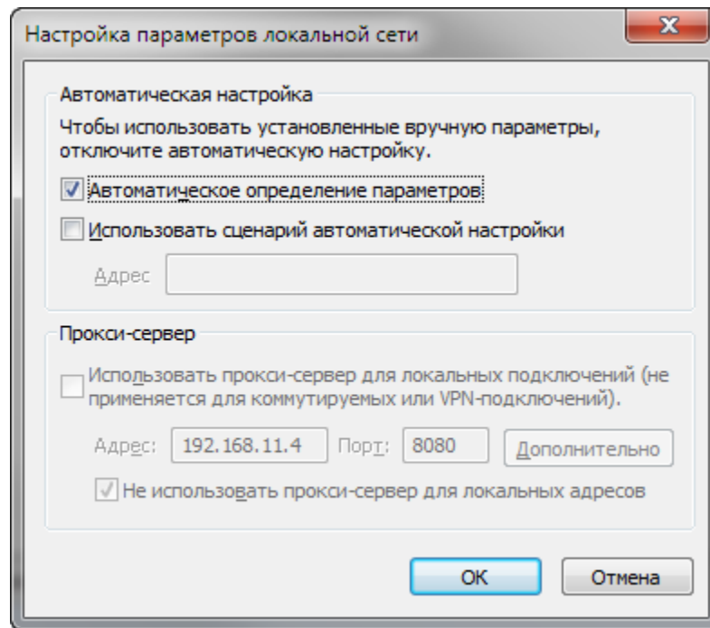
Рисунок 12. Настройка работы через прокси-сервер
