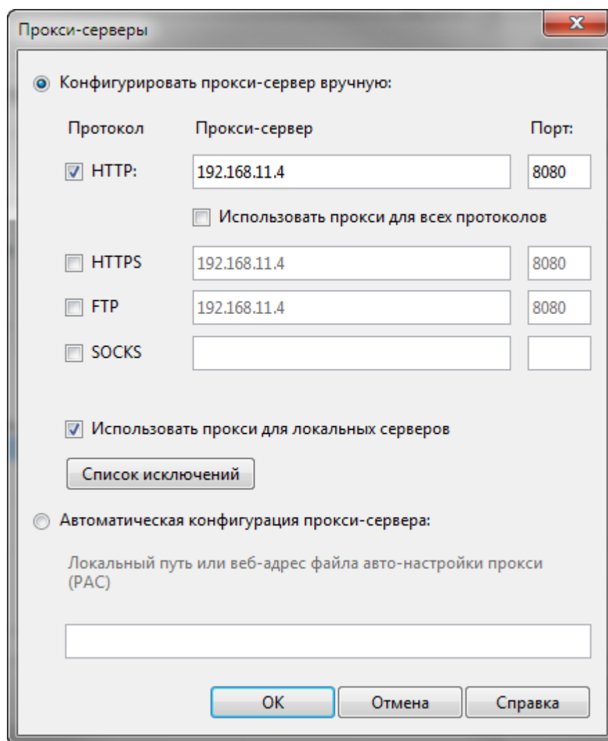
Рисунок 17. Настройка работы через прокси-сервер
